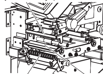
補助ローラ 印字ローラ
